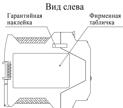
Рисунок Е.1 - БСП сигнализаторов СТМ-30М
