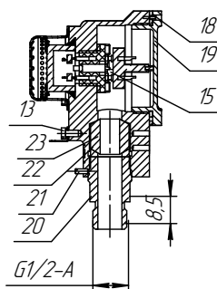
Рисунок В.4 - Датчик с разъемным соединением
