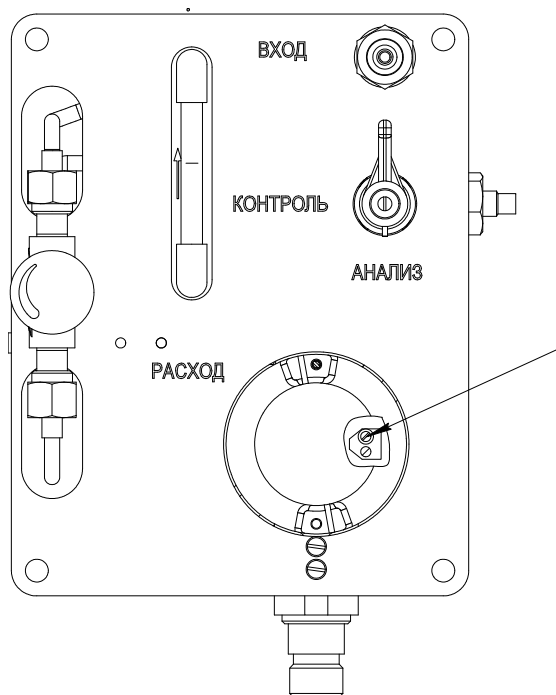
Рисунок Е.1 - БСП сигнализаторов СТМ-30М
